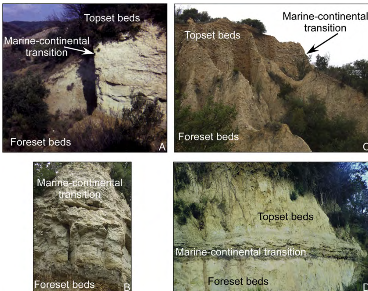
Figure 13. Examples of the marine–continental transition observed within the Zanclean Gilbert-type fan deltas near the MES. A, Poc Calbeil (Néfiach). B, Detail at Poc Calbeil (Néfiach). C, Les Escoumes (Vinça). D, Els Pontells (Vivès).
